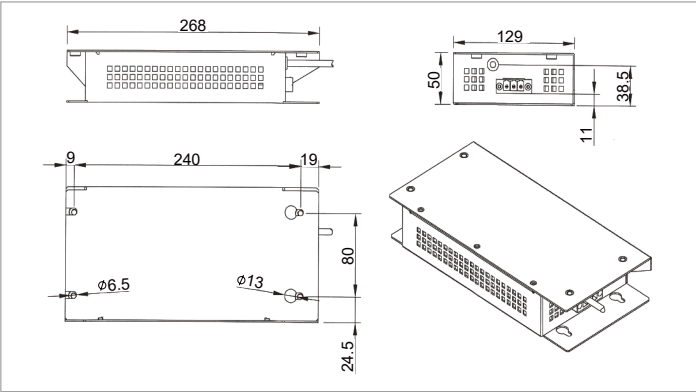
装配图中图表的详细信息不具有约束力。通用公差 DIN2768-c
