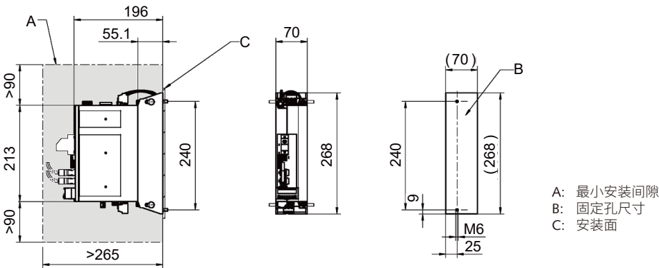
ACS1-W018/28/36 示意图（标准安装）
