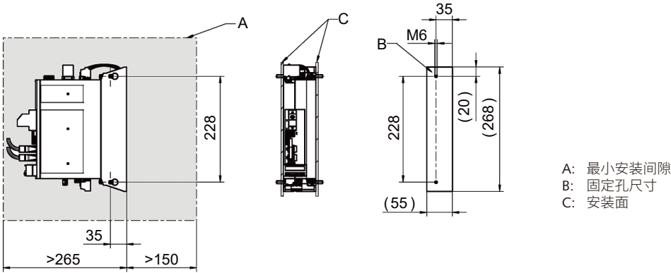
ACS1-W018/28/36 示意图（左侧或右侧安装）
