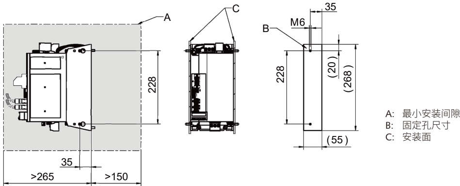
ACS1-W054 示意图（左侧或右侧安装）
