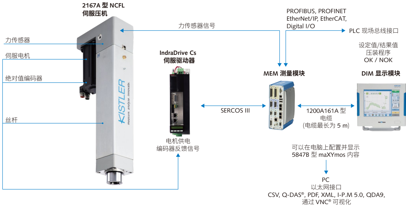
图 2: 2167A 型配 5847B 型系统原理图
