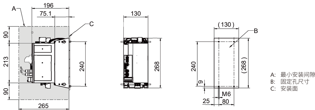
ACS1-W054 示意图（标准安装）
