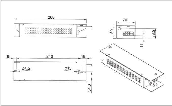
装配图中图表的详细信息不具有约束力。通用公差 DIN2768-c
